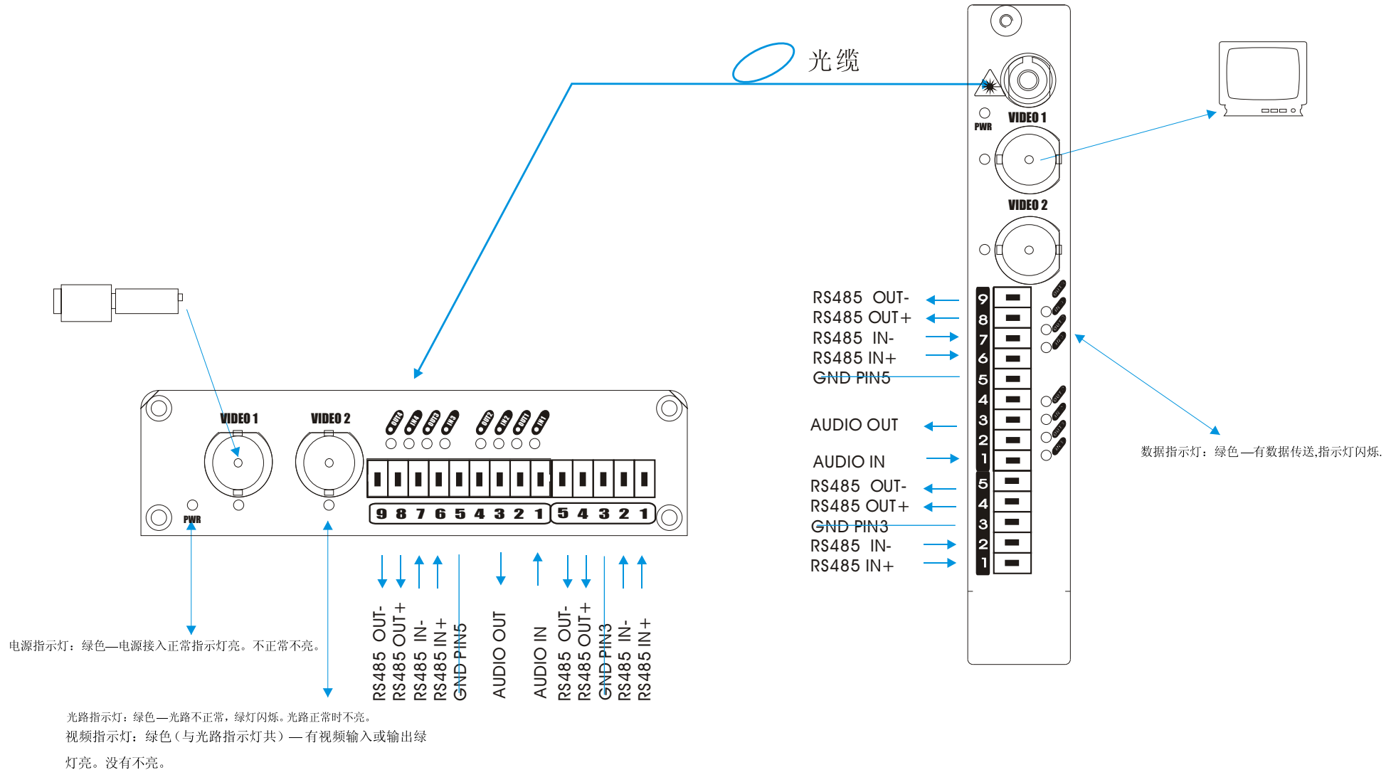
YC2033-SD-1A-2D5二路视频加二路双向RS485加一路双向对讲音频光端机接线线图
